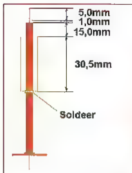
Een halve golf straler element. Hiervan zijn er 7 nodig.
